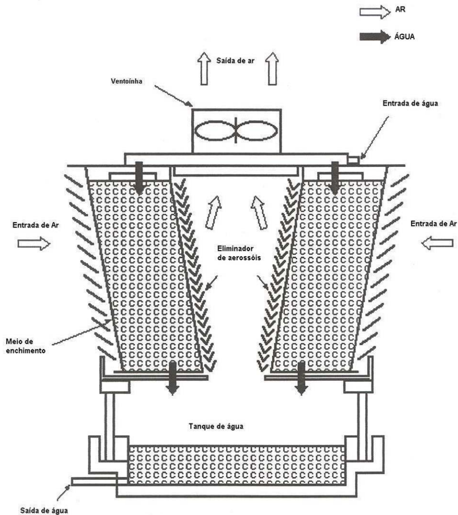
Figura 7: Torre de arrefecimento ou refrigeração para edifícios de grande dimensão (Department of Human Services "Guidelines for Controlo of Legionnaires Disease", Victoria State Austrália)
