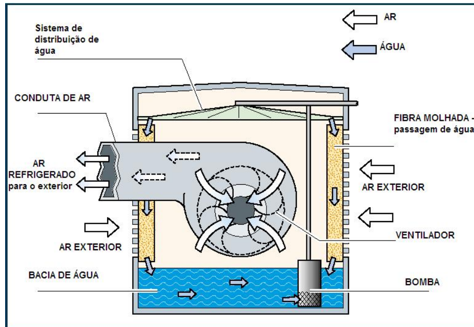
Figura 10: Exemplo de um sistema de arrefecimento por evaporação ( Department of Human Services “Guidelines for Control of Legionnaires Disease”, Victoria State Austrália)
