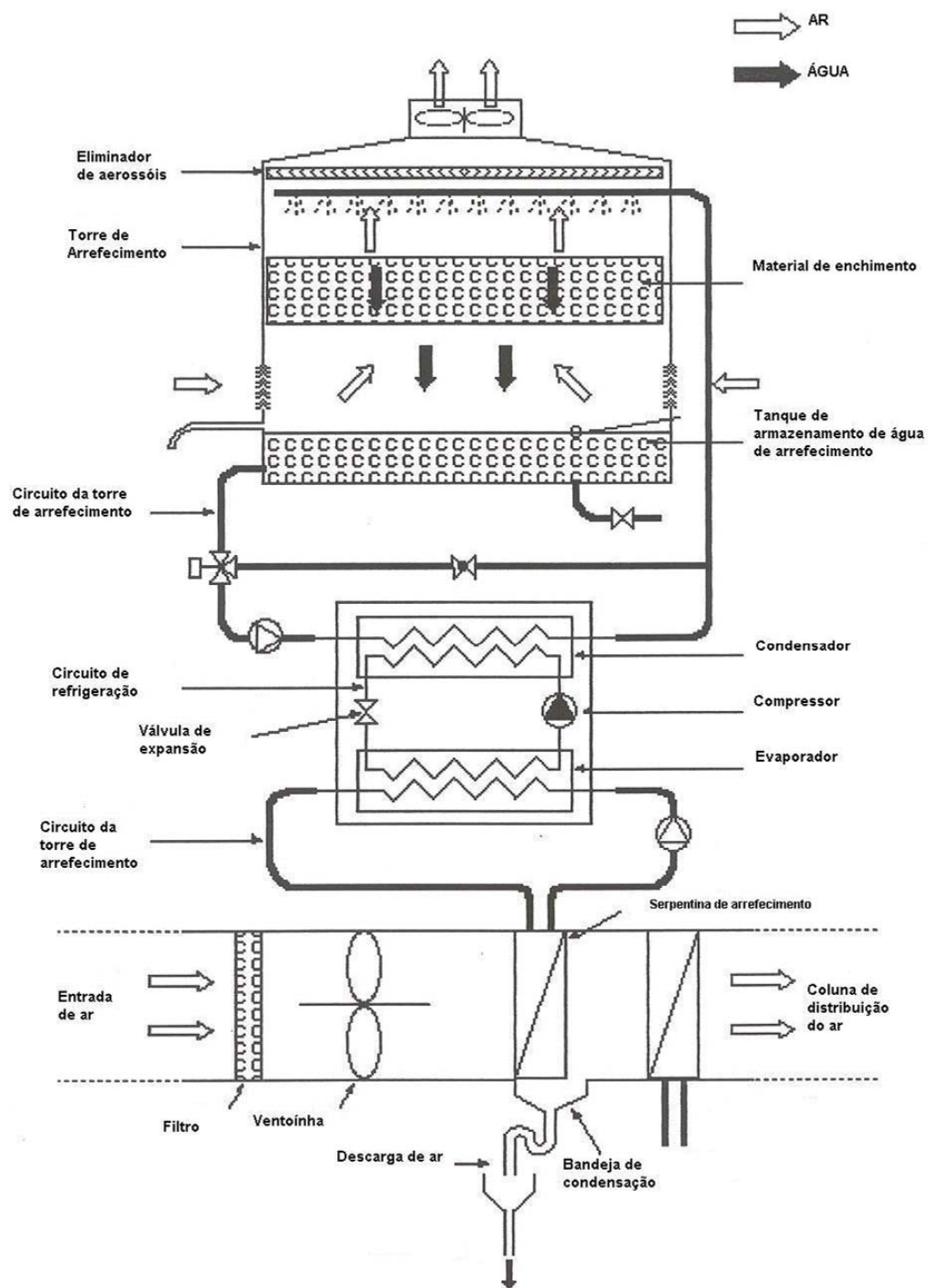
Figura 8: Sistema de ar condicionado para edifícios de grande dimensão (Department of Human Services “Guidelines for Control of Legionnaires Disease”, Victoria State Austrália)
