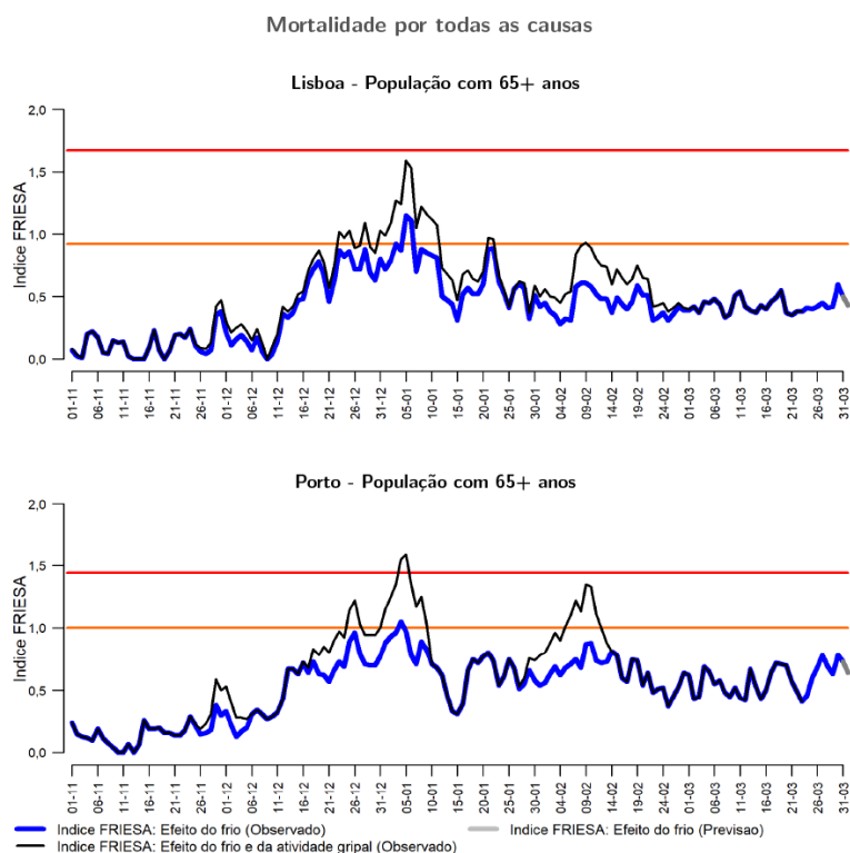
FIGURA 2. Índice FRIESA para a população com 65 ou mais anos, nos distritos de Lisboa e do Porto, a 31/03/2025 | Fontes: INSA e IPMA. Autoria: INSA
