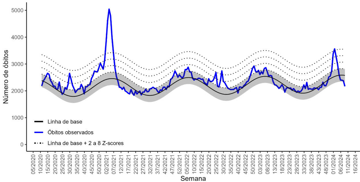
FIGURA 28. Evolução da mortalidade por todas as causas, semanal, entre 02/03/2020 e 25/02/2024. Nota: A linha azul corresponde à mortalidade observada, a linha preta à linha de base e as linhas a tracejado a desvios de 2, 4, 6 e 8 z-scores da linha de base. A área a sombreado corresponde ao corredor de valores esperados para a época do ano. | Fonte: SICO-DGS; Autoria: INSA.
