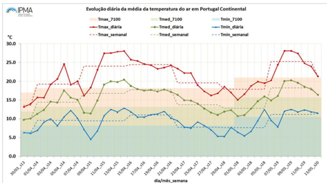
FIGURA 1. Evolução diária das temperaturas mínimas, médias e máximas do ar em Portugal Continental | Fonte e Autoria: IPMA
