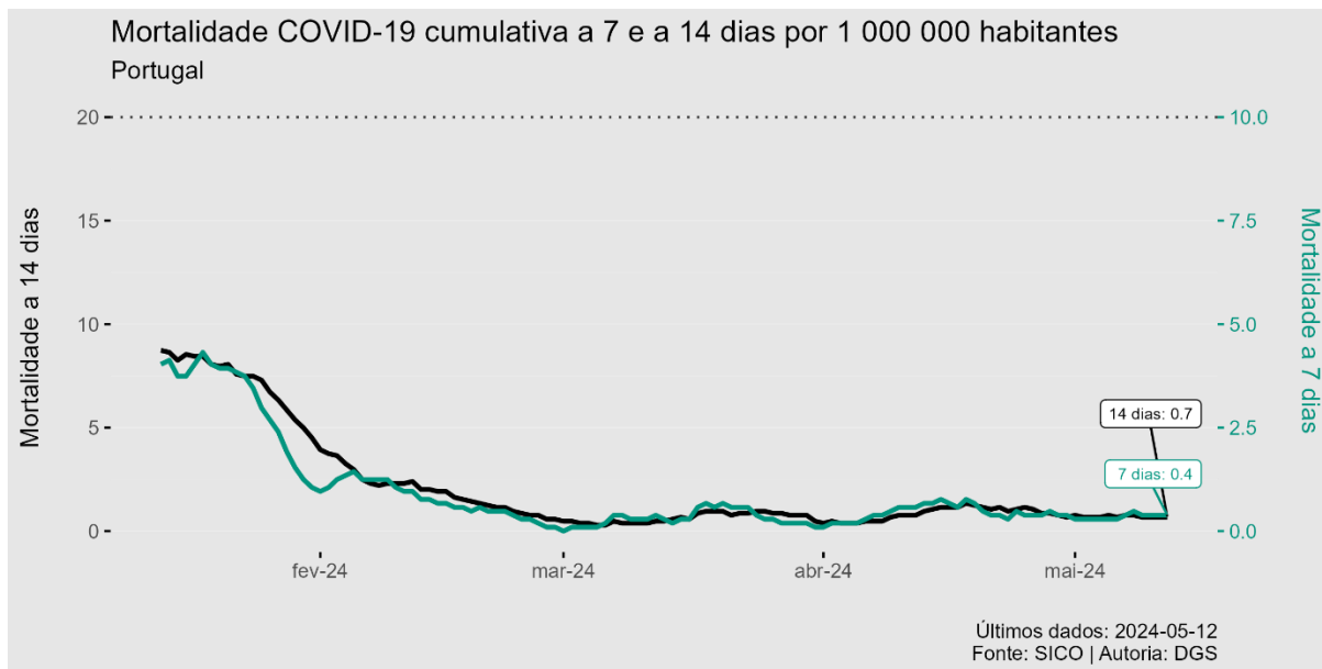
FIGURA 19. Mortalidade por COVID-19 (acumulada a 14 dias e a 7 dias por 1 000 000 habitantes) até 12/05/2024, Portugal | Fonte: SICO-DGS. Autoria: DGS.
