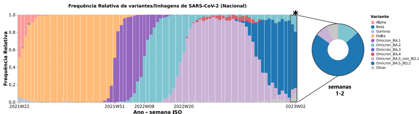
FIGURA 10: Evolução da frequência relativa semanal das variantes de SARS-CoV-2 em circulação em Portugal entre as semanas ISO 22 (31/05/2021 a 06/06/2021) e 2 (09/01/2023 a 15/01/2023). | Fonte: INSA. Autoria: INSA
