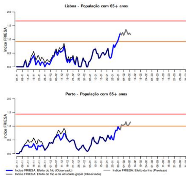
FIGURA 2: Índice FRIESA para a população com 65 ou mais anos, nos distritos de Lisboa e do Porto, a 01/02/2023. | Fontes: INSA e IPMA. Autoria: INSA
