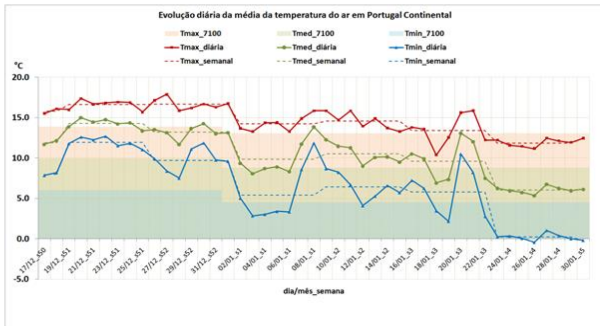
FIGURA 1: Evolução diária das temperaturas mínimas, médias e máximas do ar em Portugal Continental. | Fonte: IPMA. Autoria: IPM
